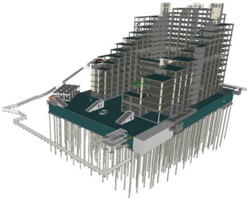
MÔ HÌNH KẾT CẤU CỦA DỰ ÁN
